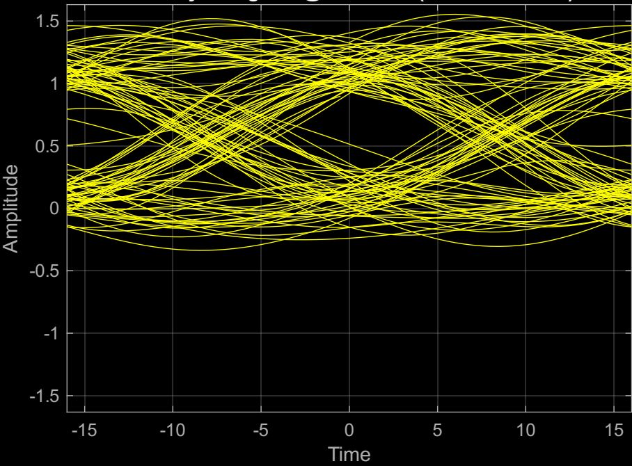
OOK Eye Diagram @ -5.0 dBm (BER \approx 1.37\text{e-}04 )
